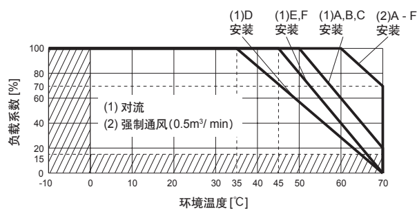
● LHA75F-12-SN, -15-SN, -24-SN, -36-SN, -48-SN 环境温度降额曲线 (参考值)
