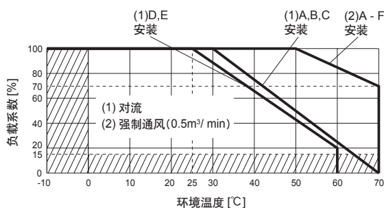
● LHA100F-5 环境温度降额曲线 (参考值)
