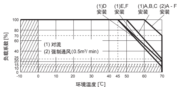
● LHA100F-12, -15, -24, -36, -48 环境温度降额曲线 (参考值)
