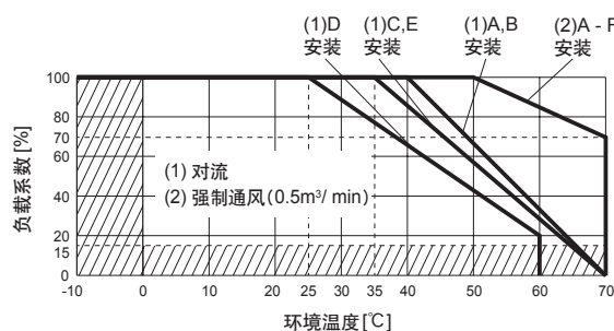
● LHA100F-12, -15, -24, -36, -48 环境温度降额曲线 (参考值)
