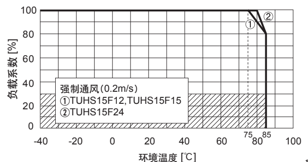
● 强制通风时TUHS15F的环境温度降额曲线 (参考值)
