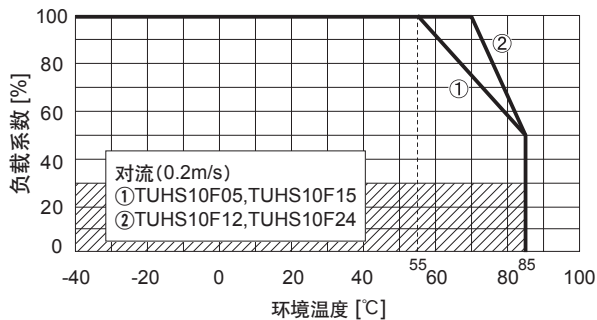
● 对流冷却时TUHS10F的环境温度降额曲线 (参考值)
