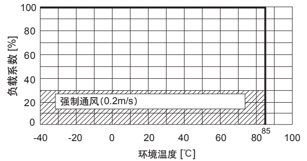
● 强制通风时TUHS5F的环境温度降额曲线 (参考值)
