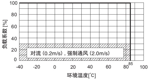
● TUHS3F的环境温度降额曲线 (参考值)
