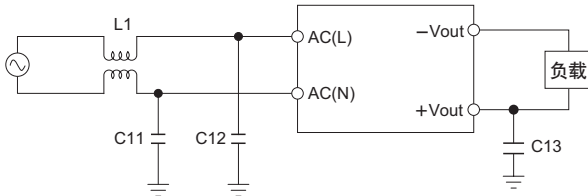
图2.2 输出端与FG连接的推荐电路
