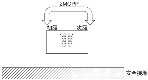
图7.1 医疗绝缘等级
