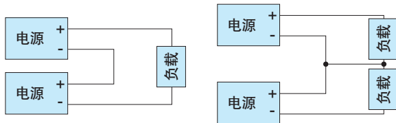
图4.1 串联运行连接示例
