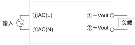
图1.1 标准应用时的连接
