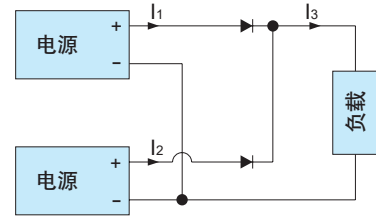
图4.2 冗余运行示例
