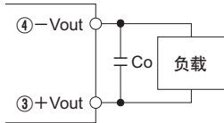
图2.1 输出端外部电容器连接示例
