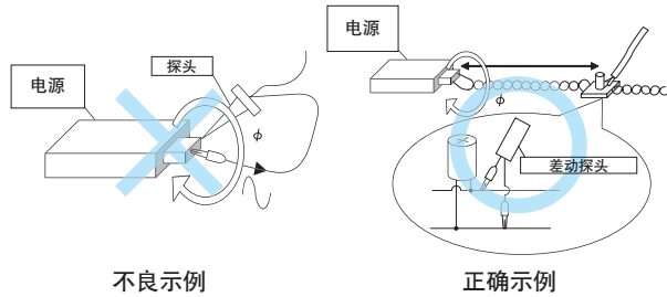
图3.2 输出纹波噪声的测量示例
