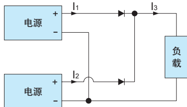
图2.2 冗余运行示例
