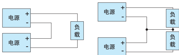
图2.1 串联运行连接示例
