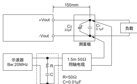
图1.1 纹波噪声的测量方法
