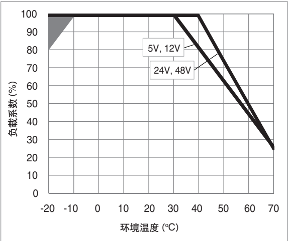
*阴影部分是电源启动时需要的降额 图1 环境温度降额曲线
