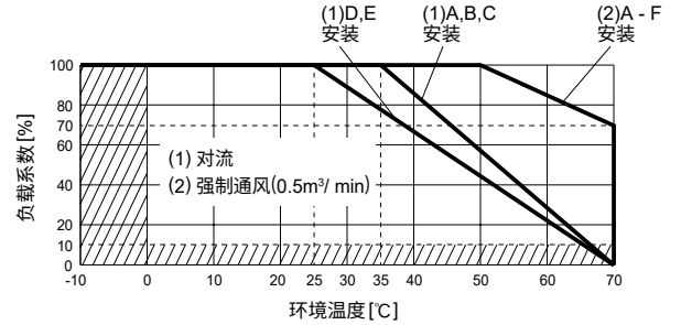
● LHA300F-24-SNY, -48-SNY 环境温度降额曲线(参考值)
