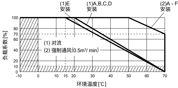
● LHA300F-12-SNY 环境温度降额曲线(参考值)
