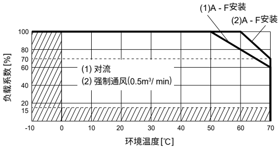
● LHA30F-3R3-SNY, -5-SN, -12-SN, -15-SN, -24-SN 环境温度降额曲线(参考值)
