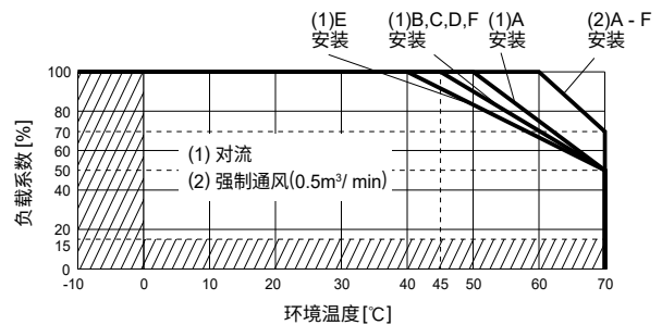
● LHA50F-12, -15 环境温度降额曲线(参考值)
