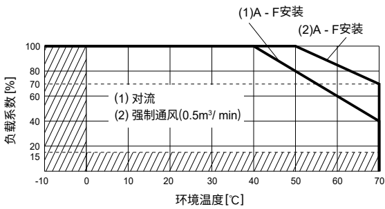
● LHA50F-3R3-Y, -5, -24, -36, -48 环境温度降额曲线(参考值)
