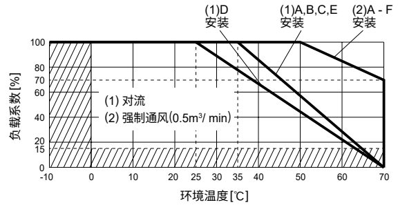
● LHA150F-24, -36, -48 环境温度降额曲线(参考值)
