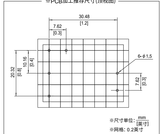
※PCB加工推荐尺寸(顶视图)
